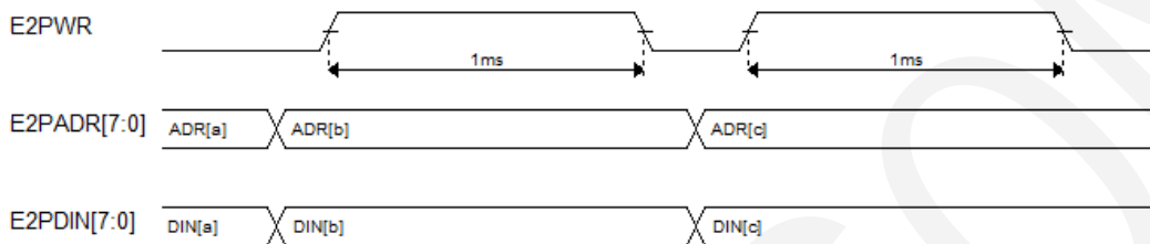
图2.9.1:内置EEPROM烧写示意图
