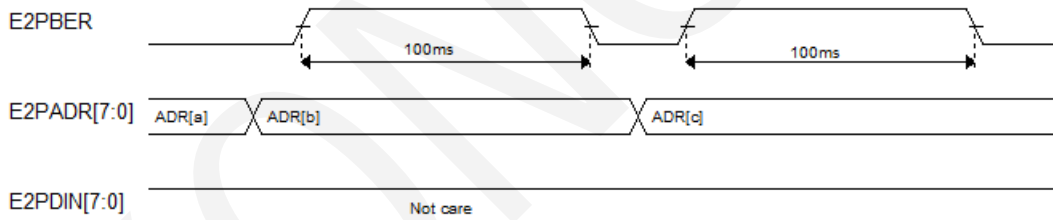
图2.9.2:内置EEPROM字节擦除示意图
