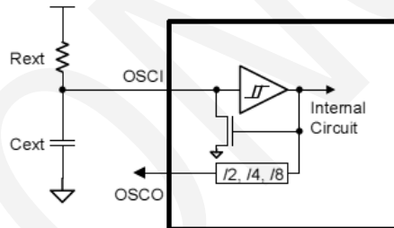
图2.11: ERC/ERIC 振荡器模式 (外部电阻电容振荡器)
