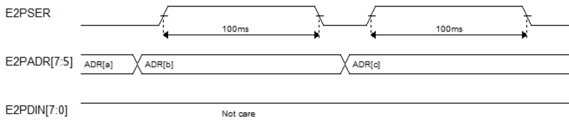
图2.9.3:内置EEPROM扇区擦除示意图
