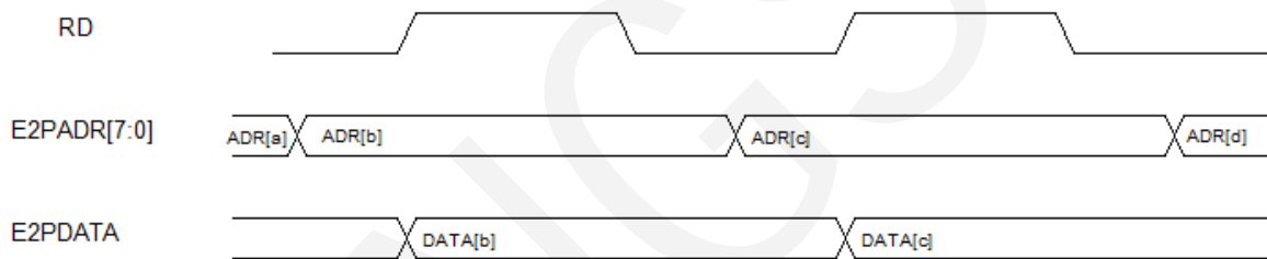
图2.9.5:内置EEPROM读操作示意图
