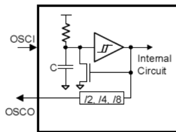
图2.12: IRC 振荡器模式 (内部电阻电容 振荡器)
