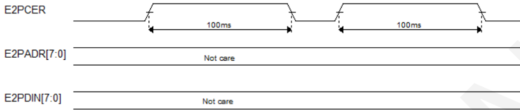
图2.9.4:内置EEPROM片擦除示意图
